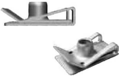
Porca rápida Citroen/Peugeot/Ford/ BMW/Mercedes/Fiat M6 x 16 x 25mm
